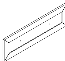
15 (679X203X15mm)x5
